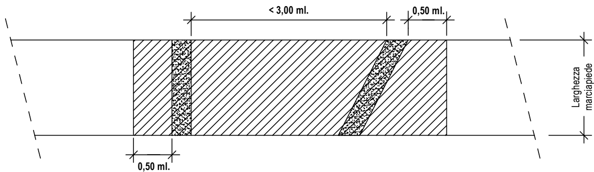
Scavo obliquo e/o trasversale all'asse del marciapiede
