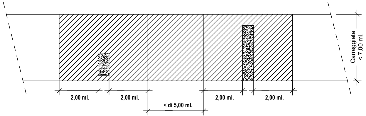
Scavi multipli trasversali all'asse della strada
