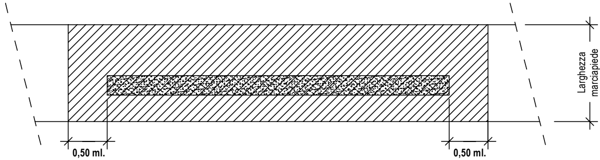
Scavo parallelo all'asse del marciapiede
