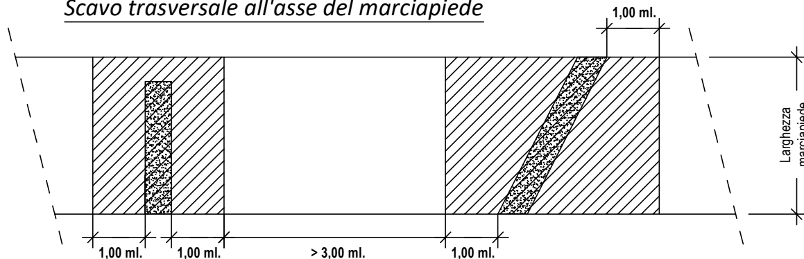
Scavo trasversale all'asse del marciapiede
