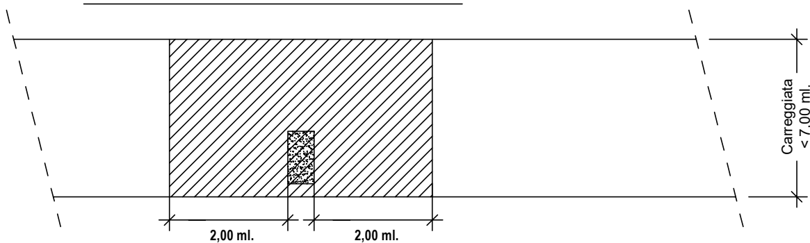
Scavo trasversale all'asse della strada
