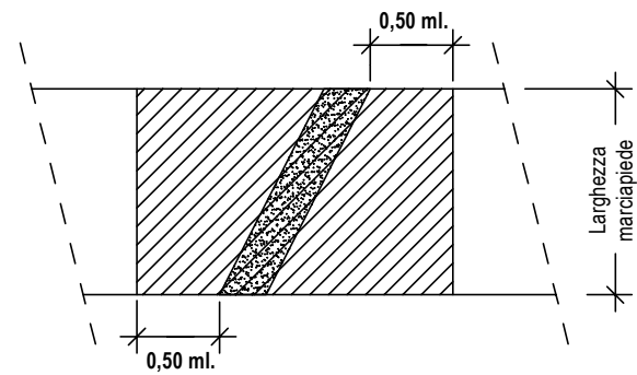
Scavo obliquo all'asse del marciapiede
