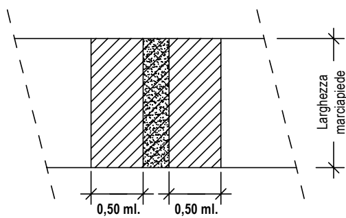
Scavo trasversale all'asse del marciapiede
